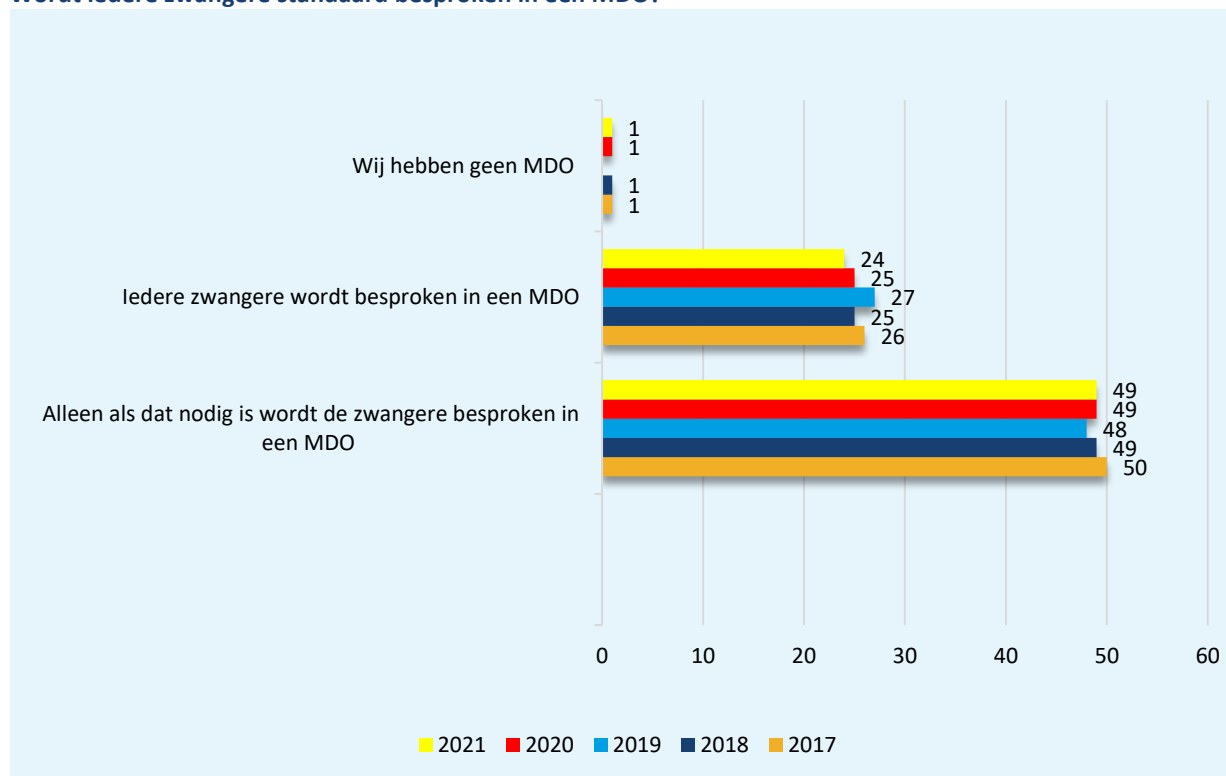
Fig. 4 MDO 2017-2021
