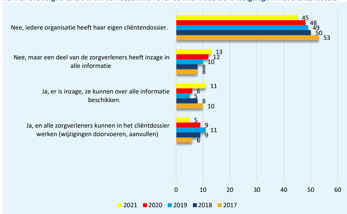
Fig. 4 MDO 2017-2021
